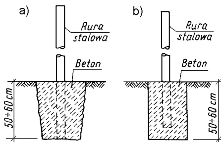
Rys. 3. Przykłady osadzenia słupków stalowych ogrodzenia w gruncie (wg [6]) 1. Słupek osadzony w betonie ułożonym bezpośrednio w dołku 2. Słupek osadzony w dołku po uprzednim oprawieniu go w bloczek betonowy
