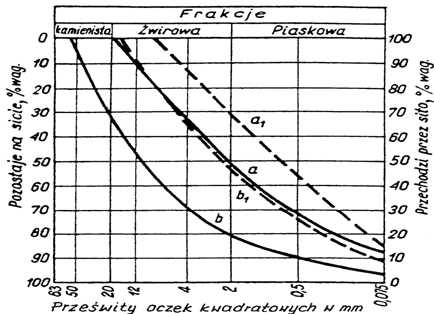
Rysunek 1. Obszar uziarnienia optymalnych mieszank żwirowych
